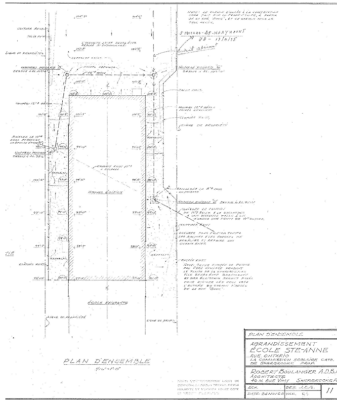
Détail du plan d'implantation de l'agrandissement de l'école Sainte-Anne, novembre 1960. (P-029-001-028, FC.18 Plans des établissements de la CSRS)
