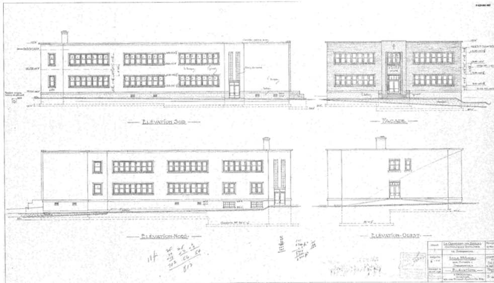
Plan des élévations de l'école Sainte-Anne, novembre 1956. (P-029-001-005, FC.18 Plans des établissements de la CSRS)
